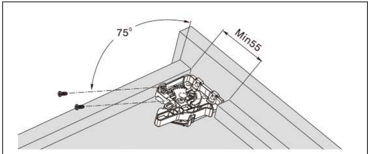
Posição dos Parafusos do Deslizamento
