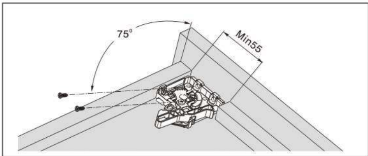
Posição dos Parafusos do Deslizamento
