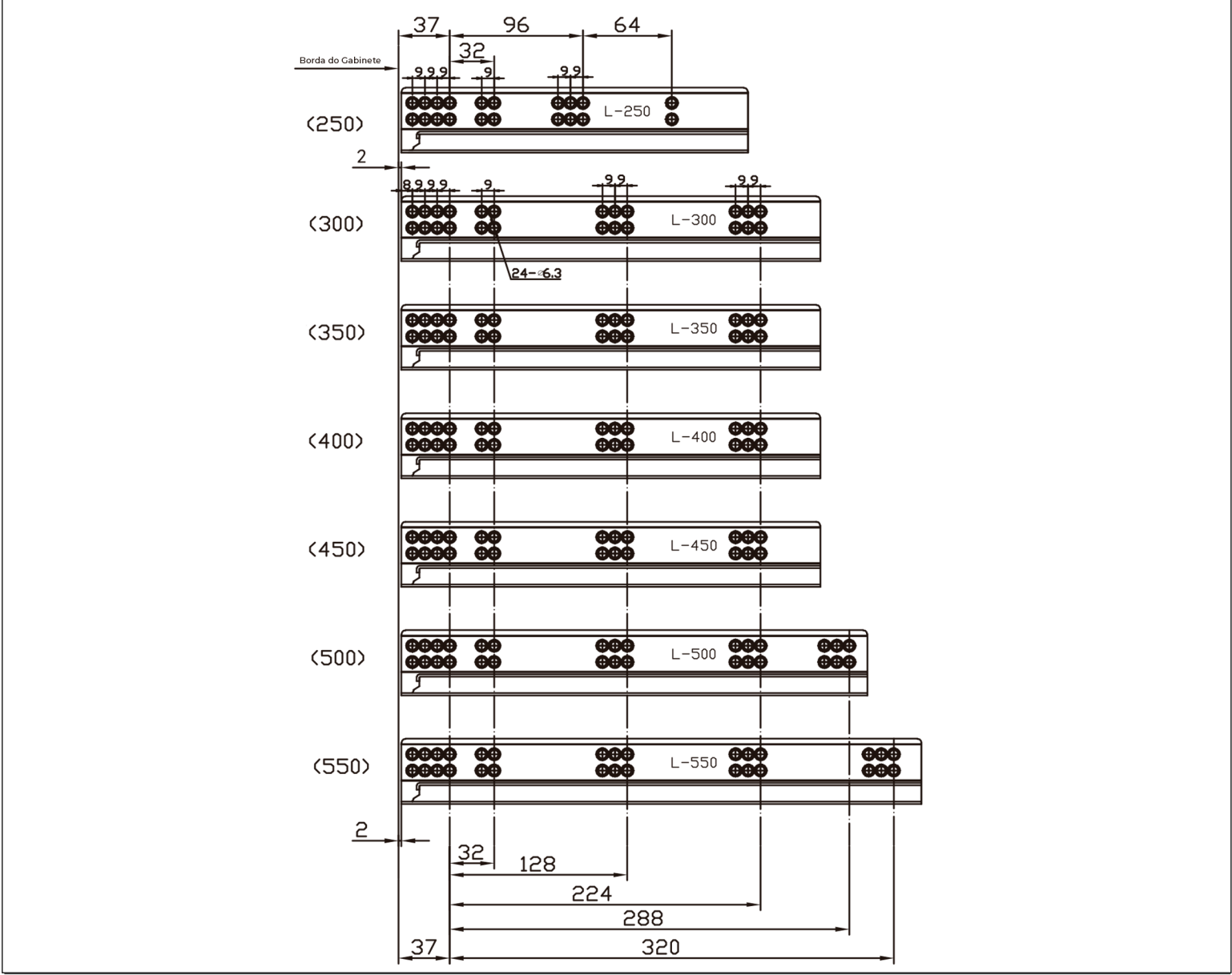
Posição dos Parafusos do Deslizamento
