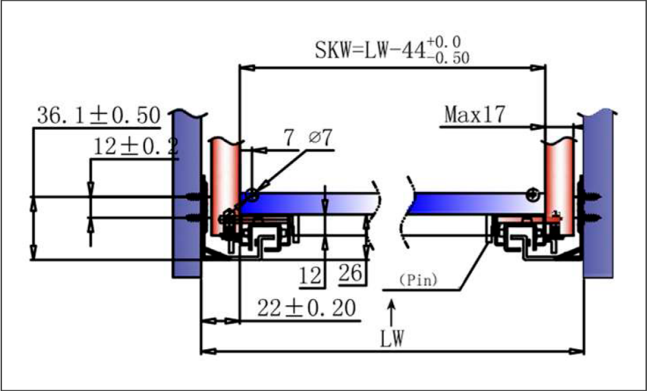
Dimensões de instalação em gaveta
